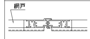
上部引違サッシ部 平面詳細図
