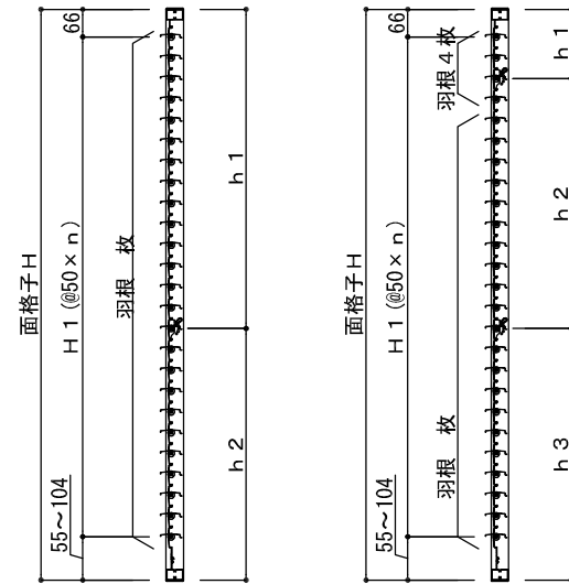
羽根可動1段
