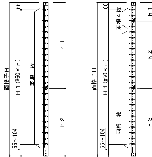
羽根可動1段
