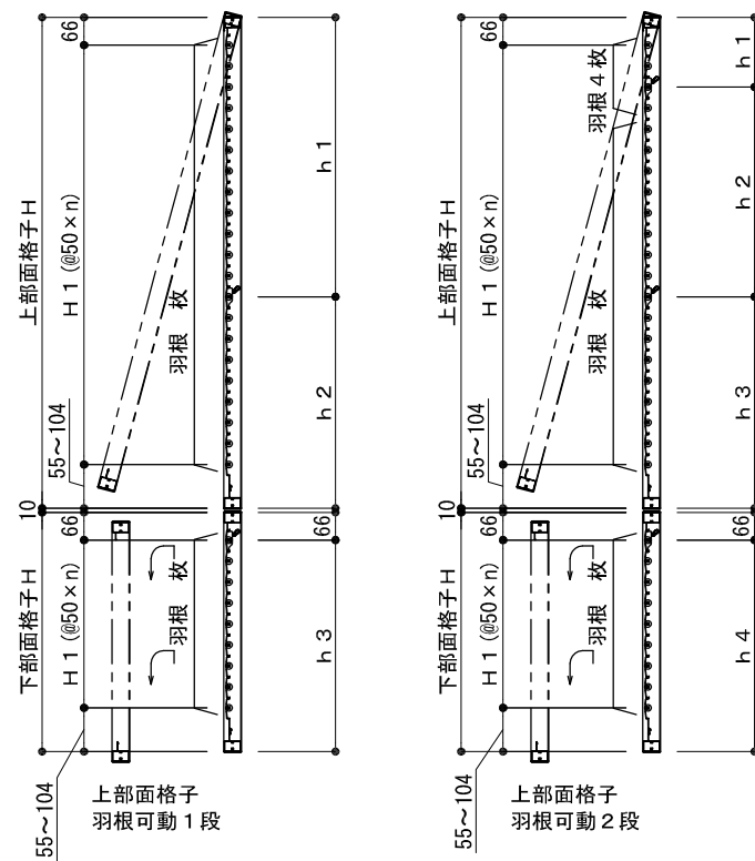
外観姿図
