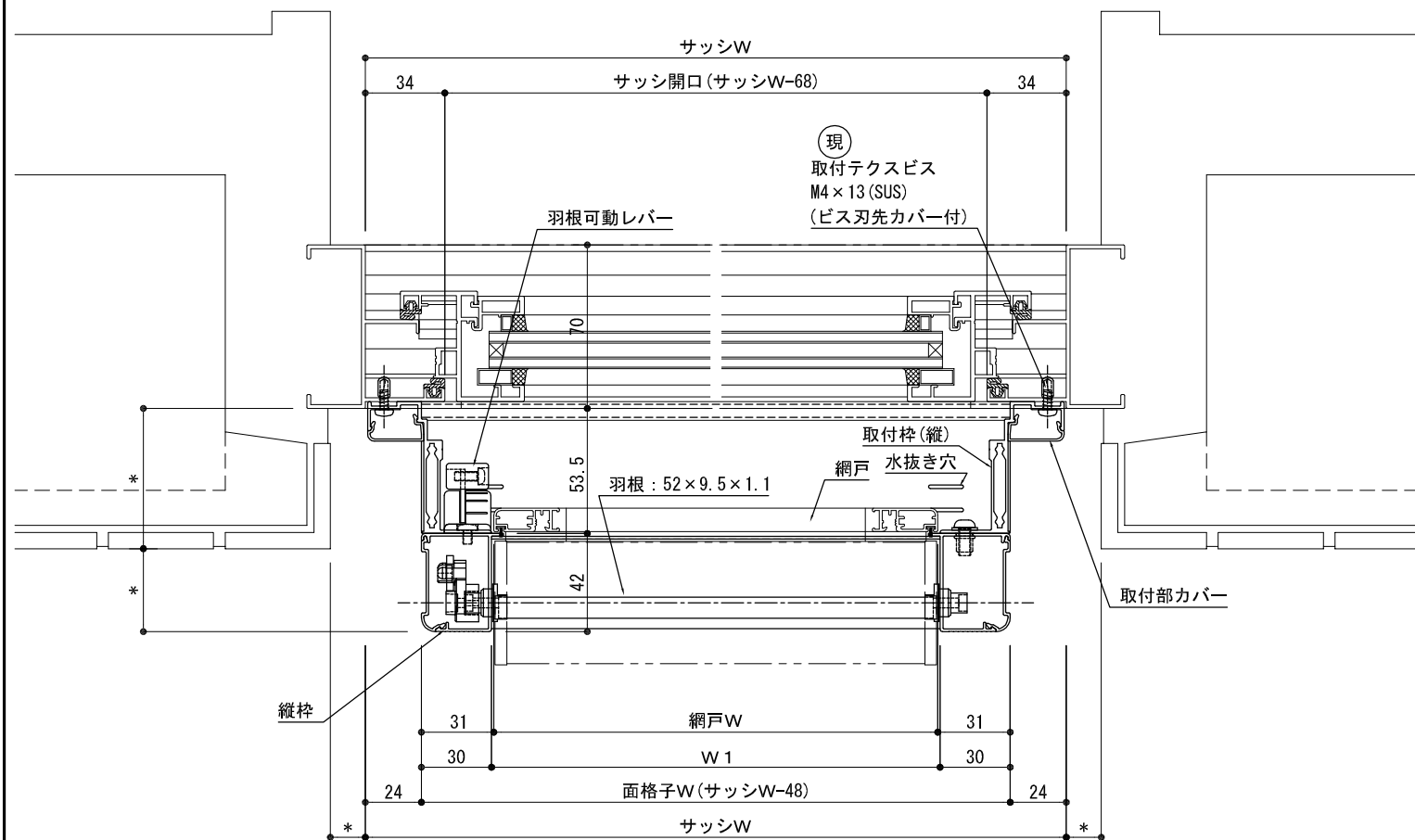
平面詳細図
