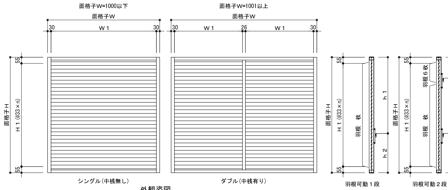
外観姿図
