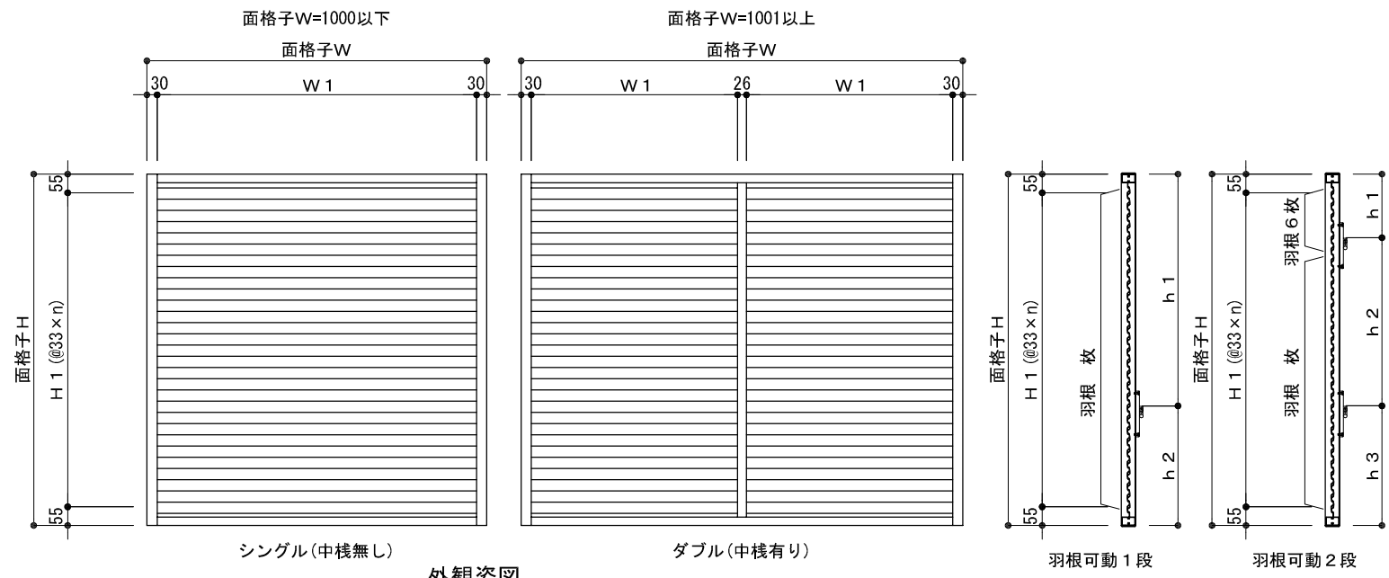
外観姿図
