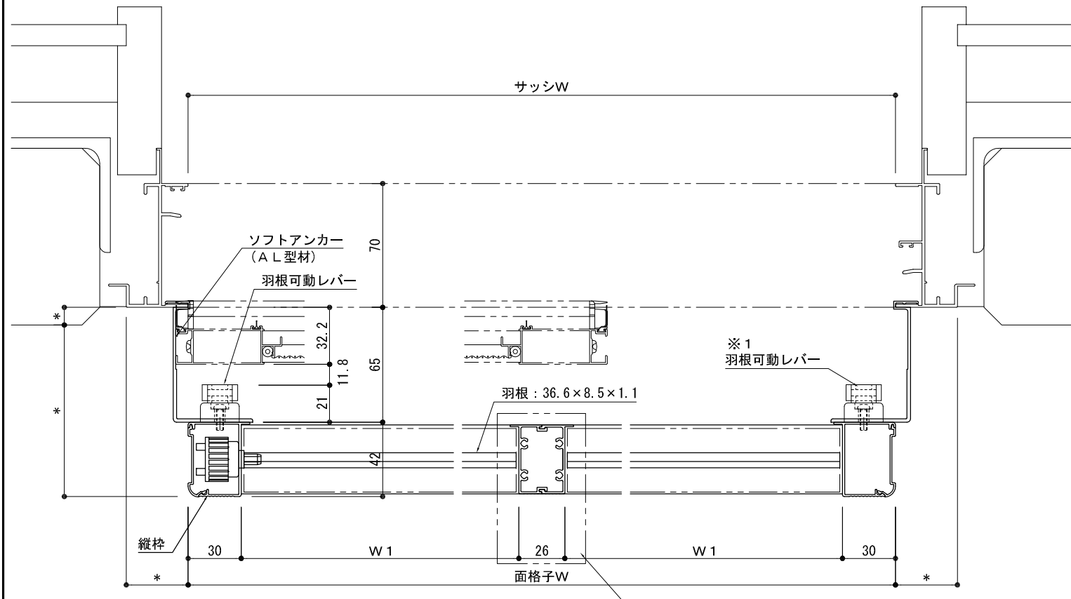
平面詳細図
