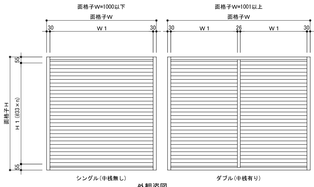
外観姿図
