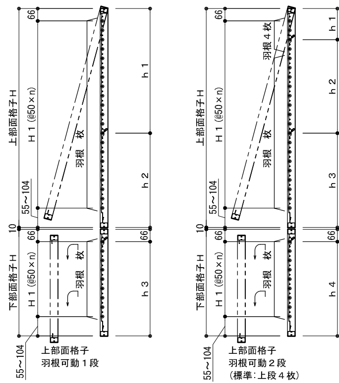
外観姿図
