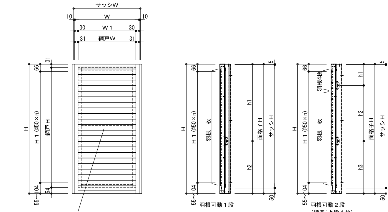
外観姿図
