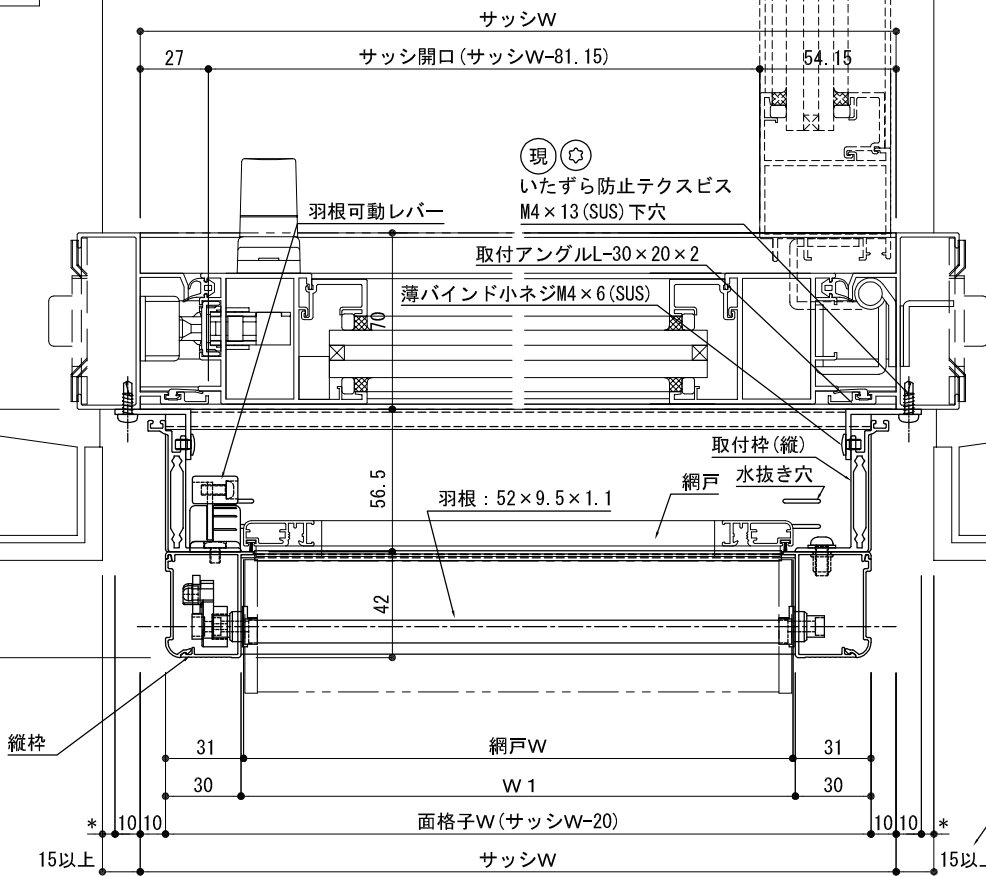
平面詳細図
