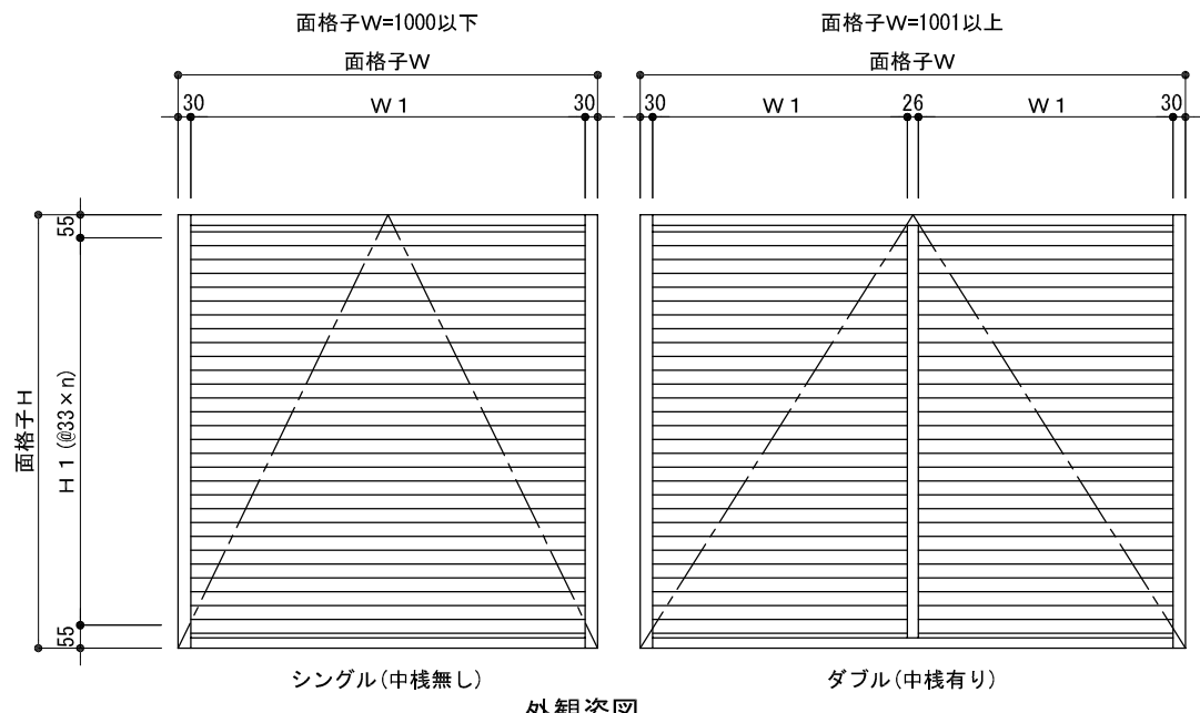
外觀姿図
