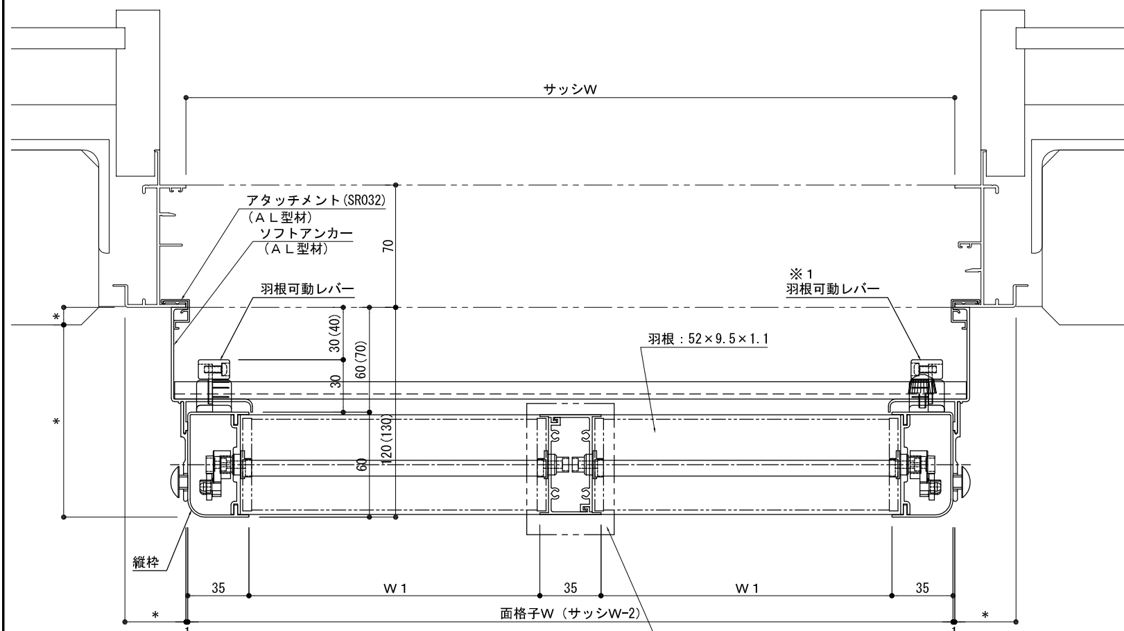
平面詳細図
