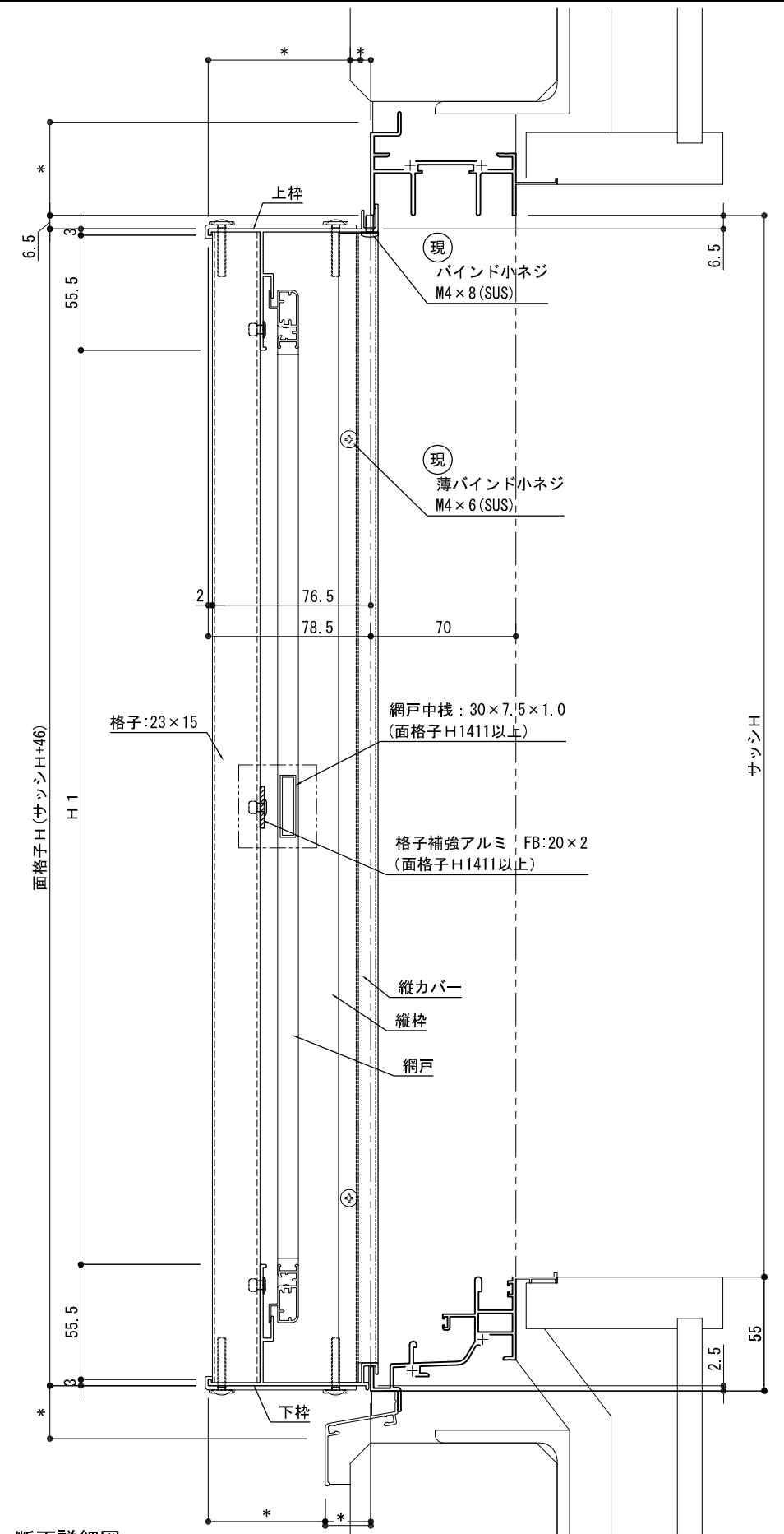
断面詳細図
