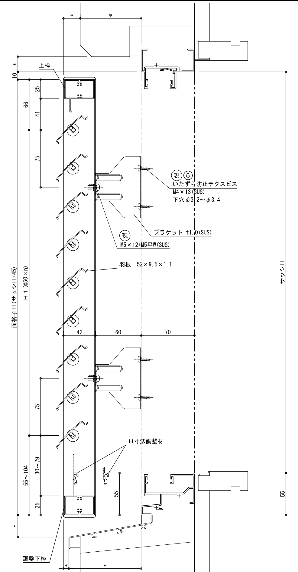
断面詳細図
