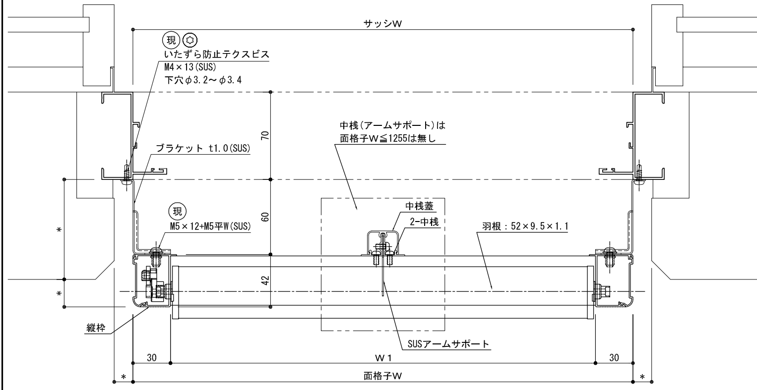
平面詳細図
