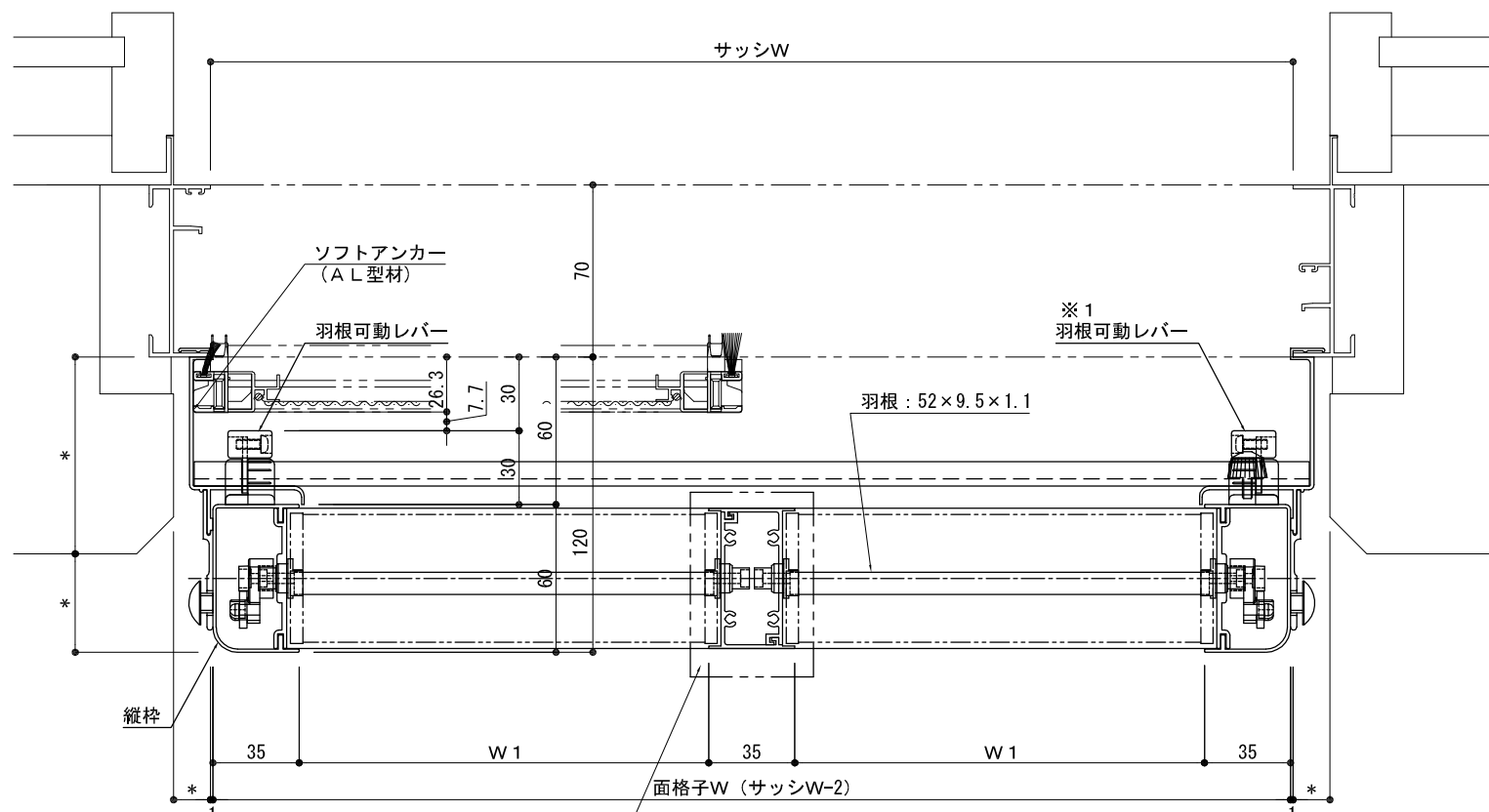
平面詳細図
