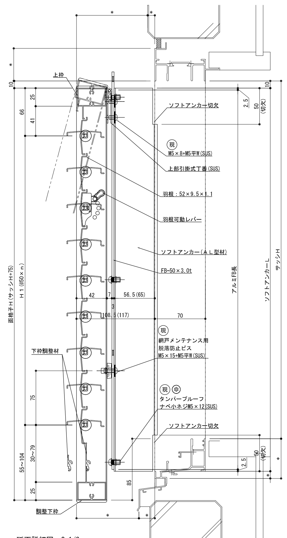
断面詳細図 S=1/3
