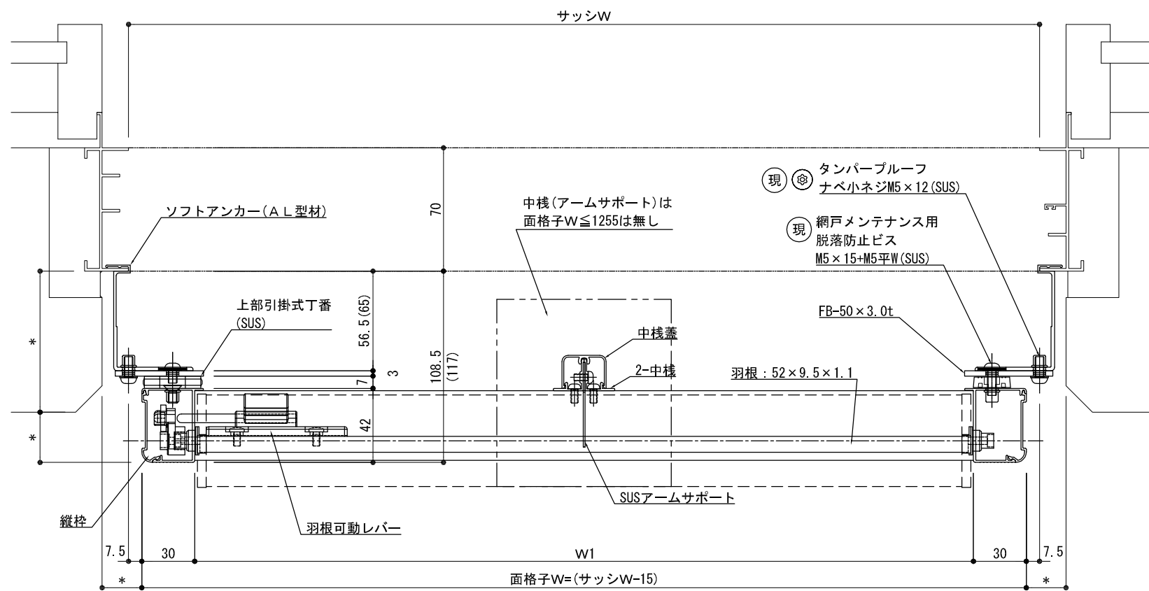
平面詳細図 S=1/3
