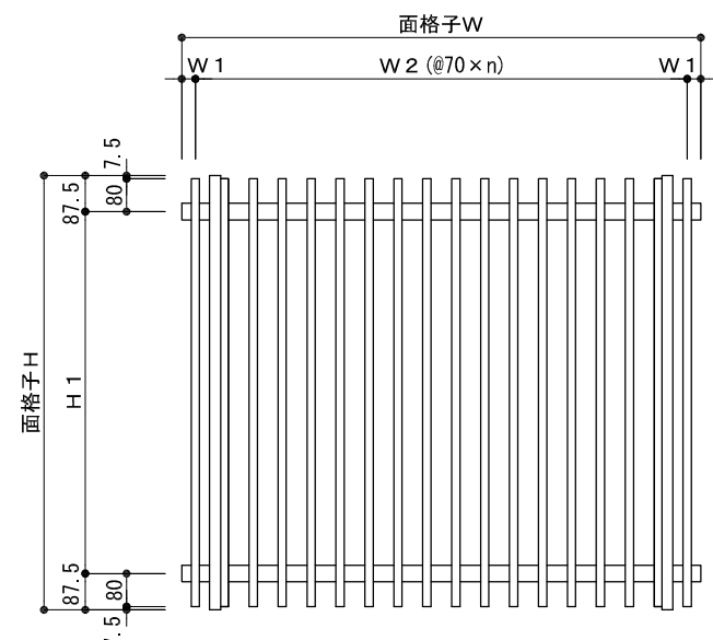
外観姿図
