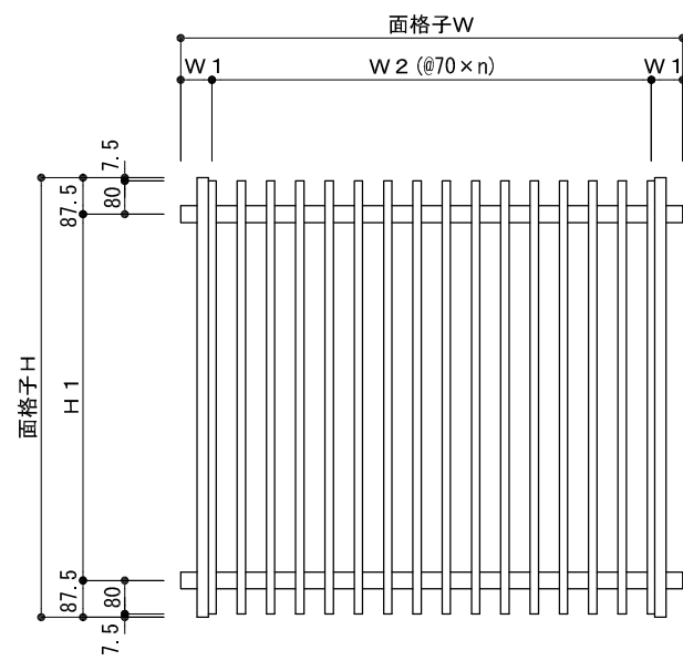
外観姿図
