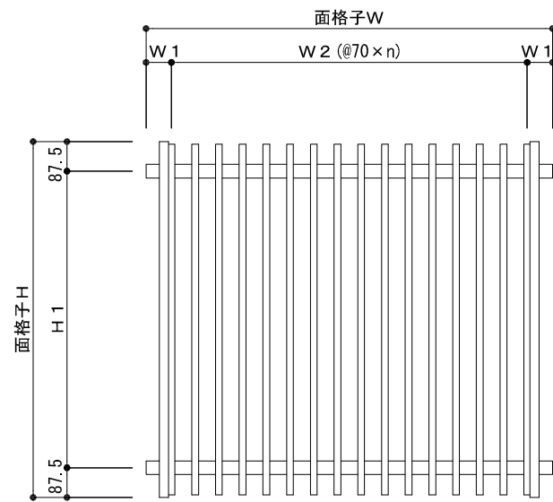
外観姿図
