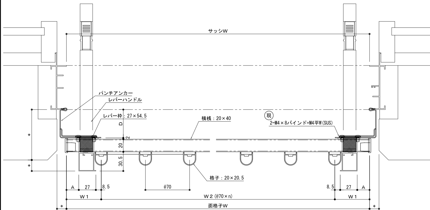
平面詳細図
