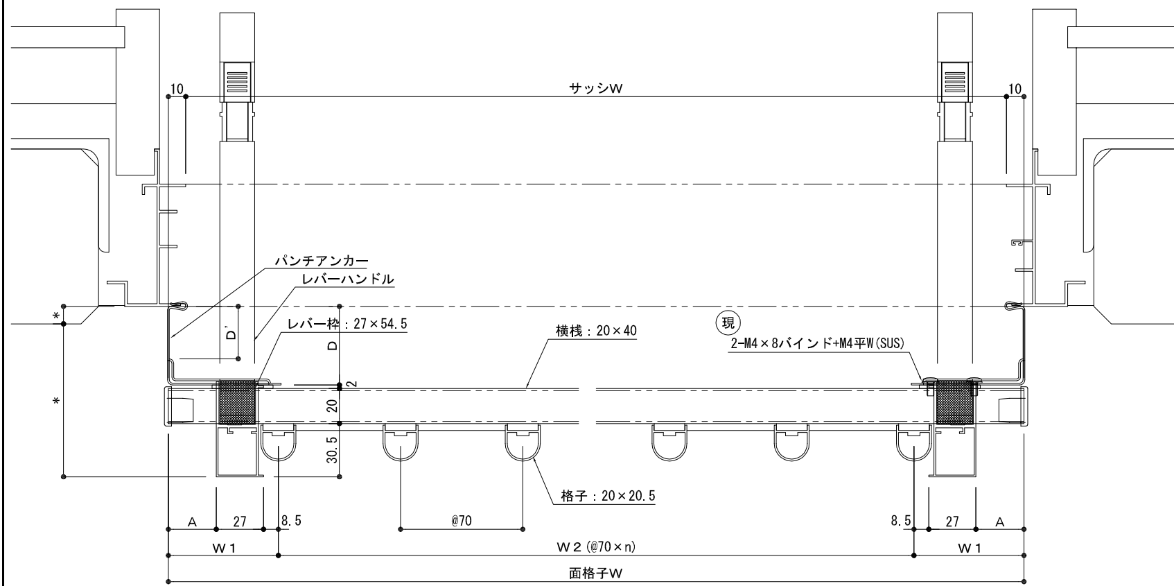
平面詳細図
