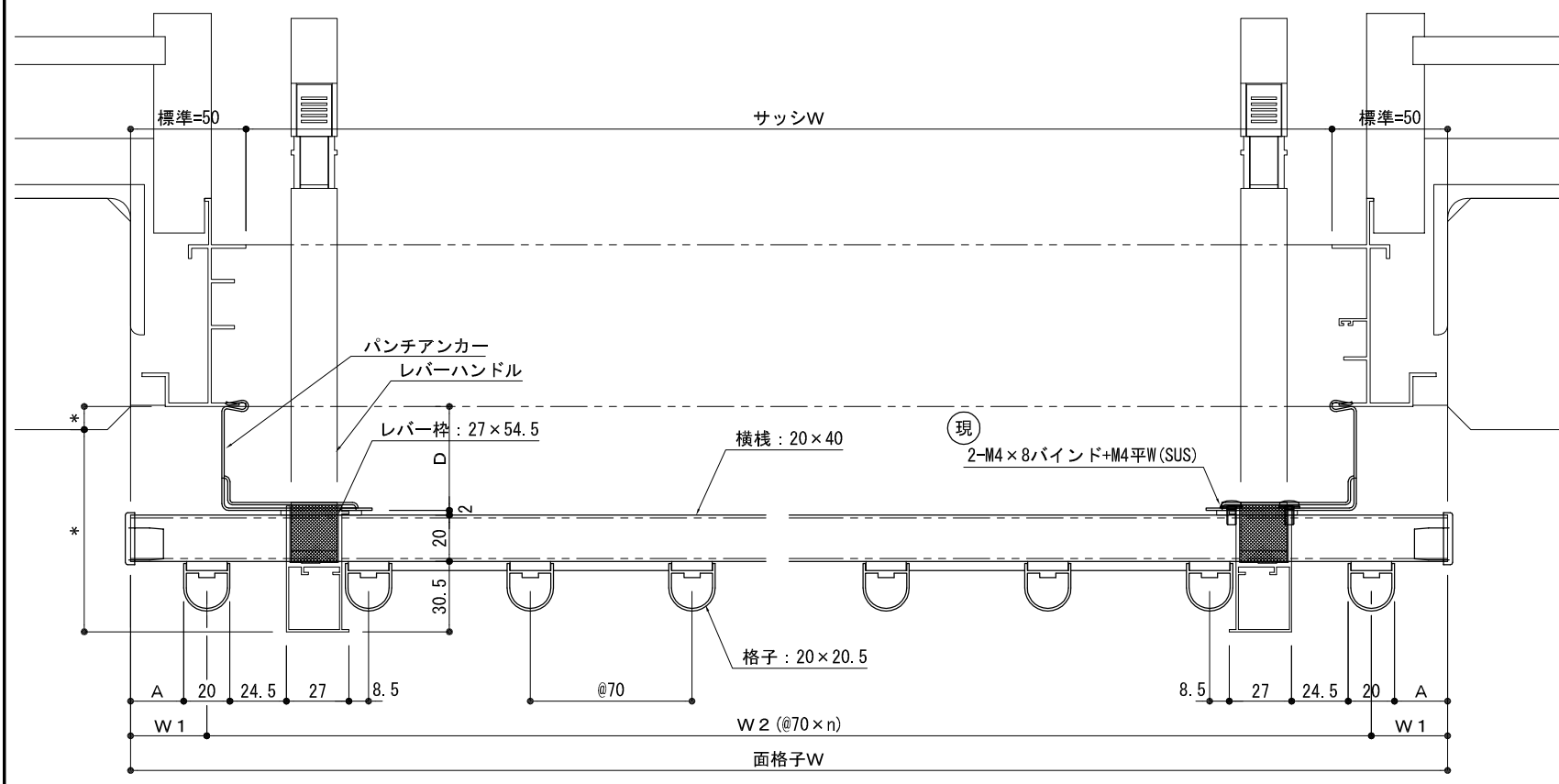
平面詳細図
