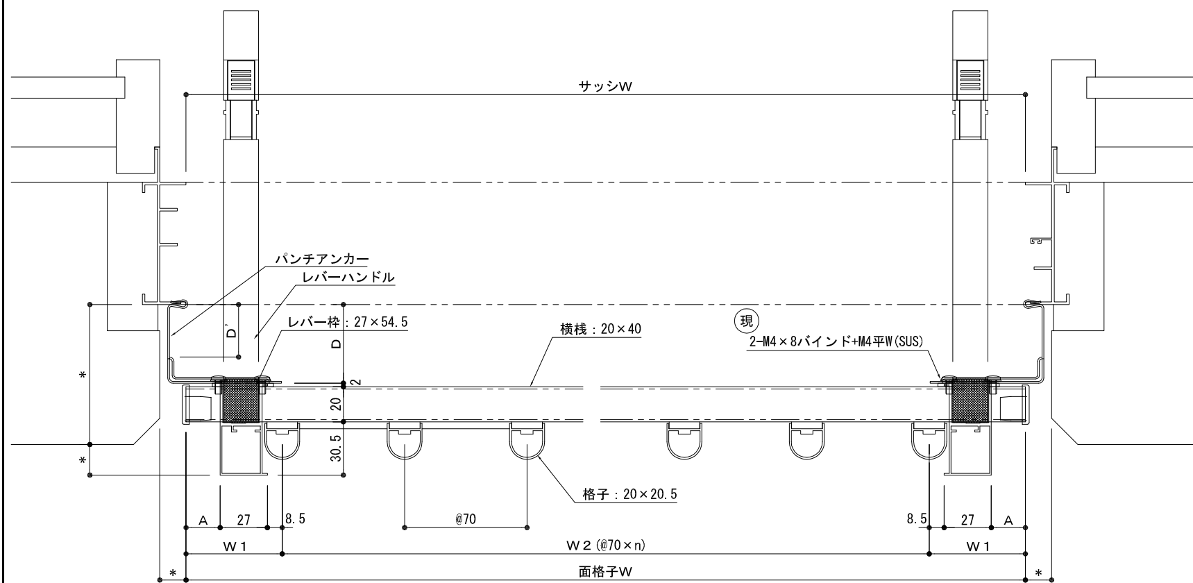
平面詳細図
