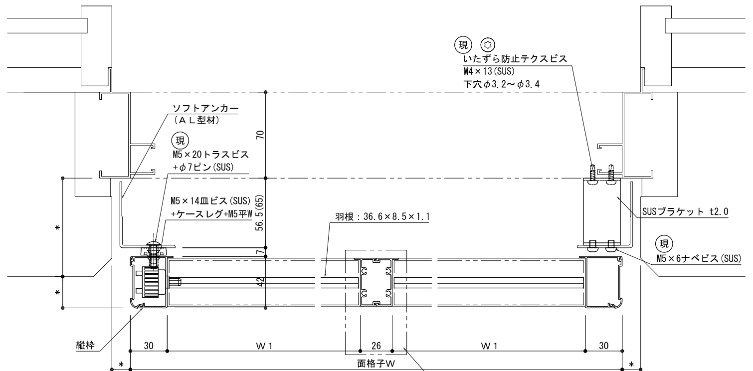
下部FIXサッシ部平面詳細図
