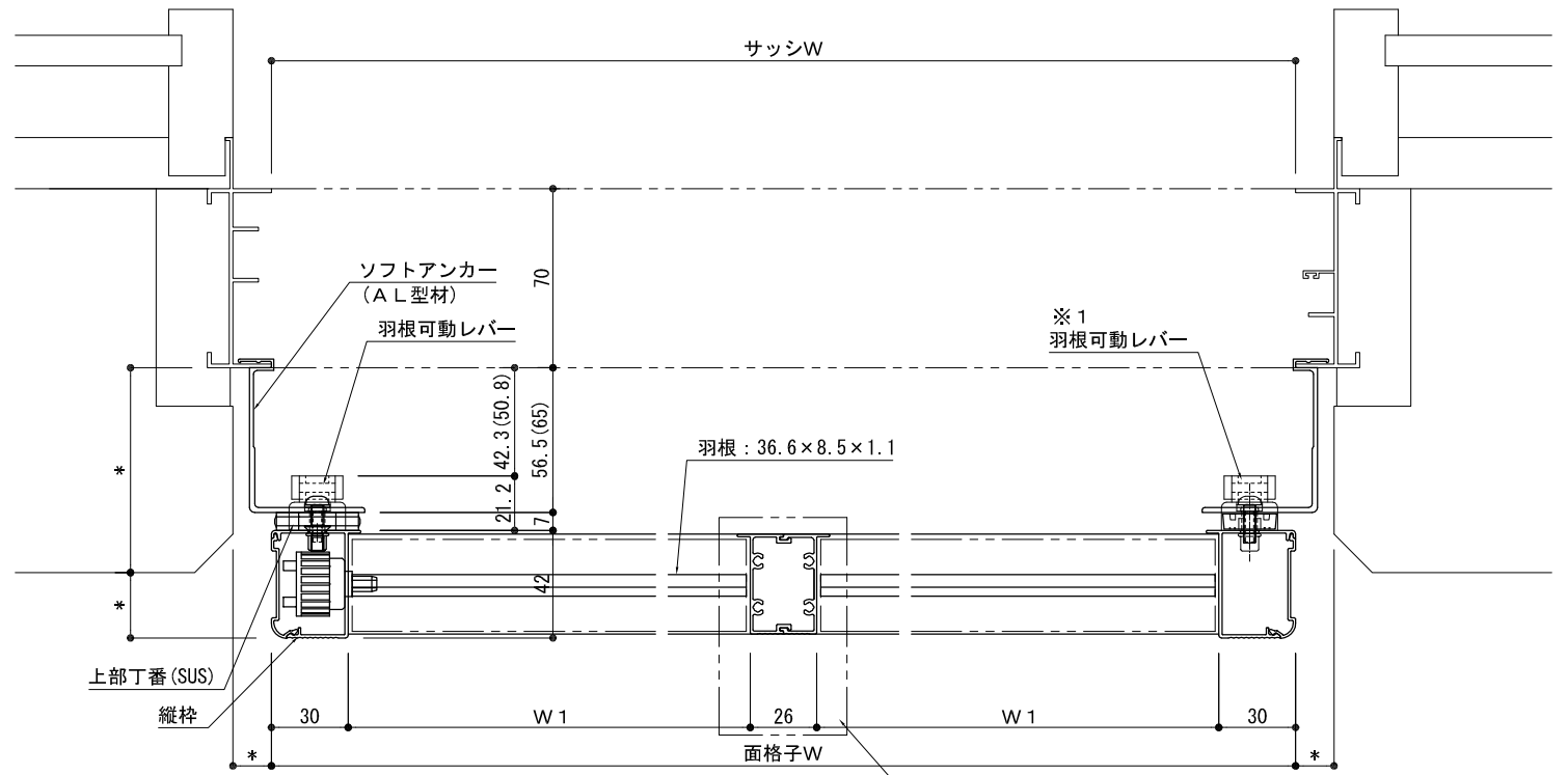
上部引違サッシ部平面詳細図
