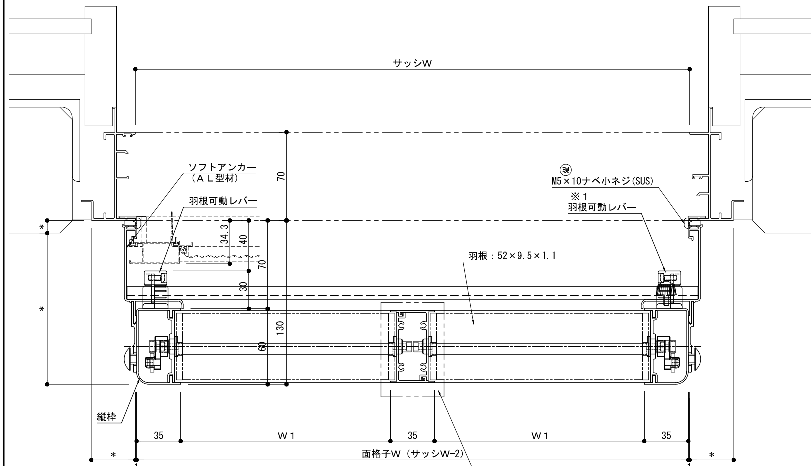
平面詳細図
