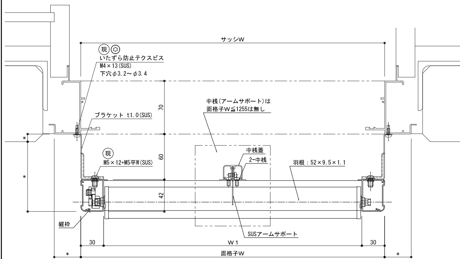
平面詳細図
