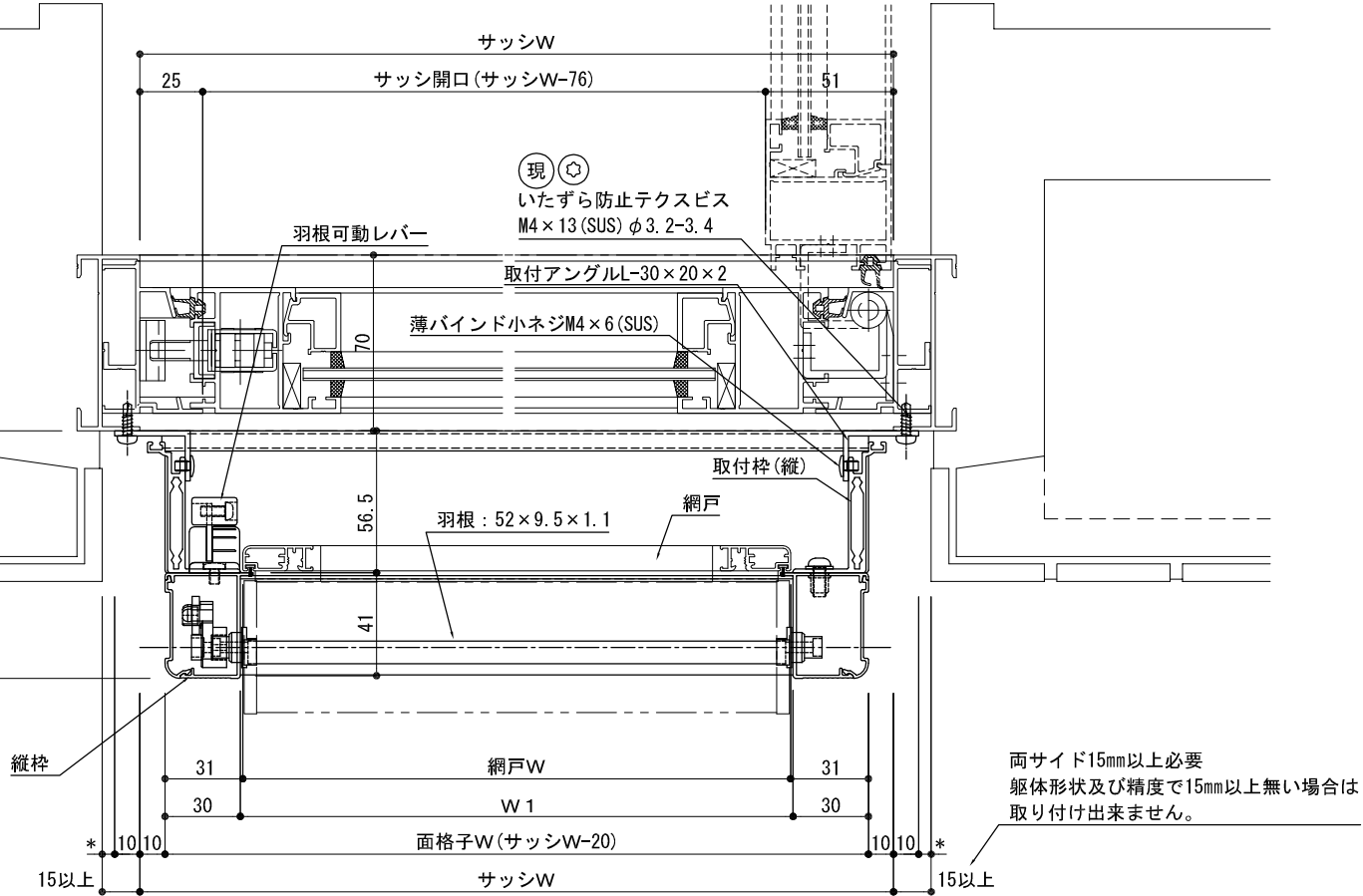
平面詳細図
