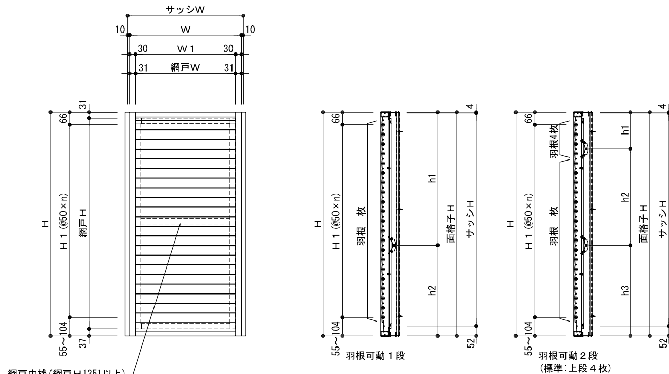
外観姿図
