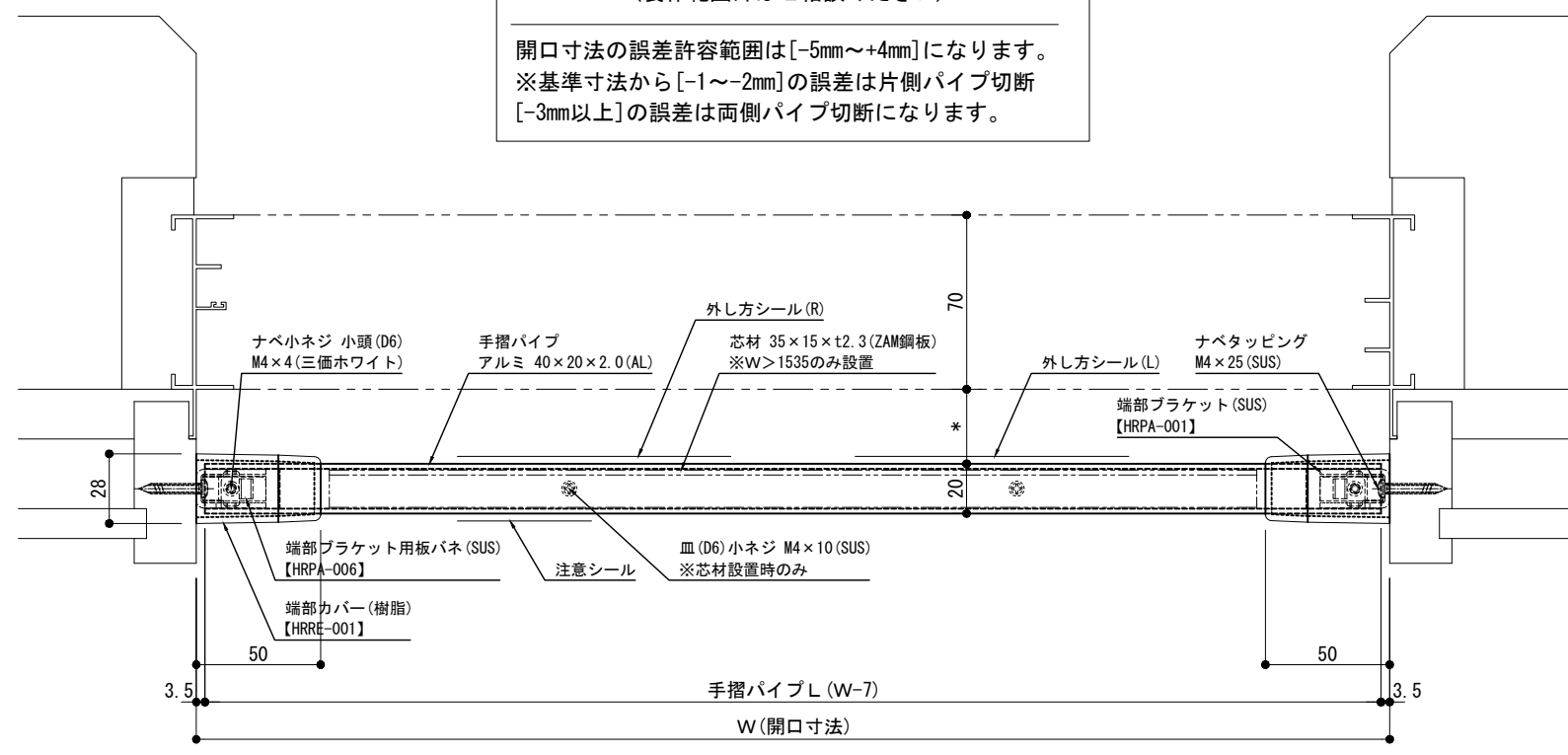
平面詳細図
