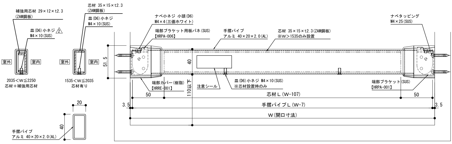
内観姿図
