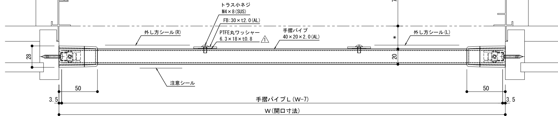
平面詳細図
